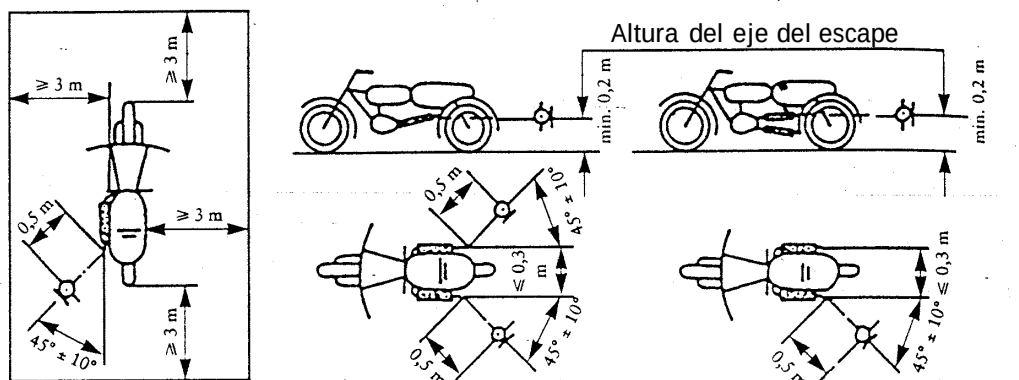
Figura 1. Croquis de posicionamiento del sonómetro 1
